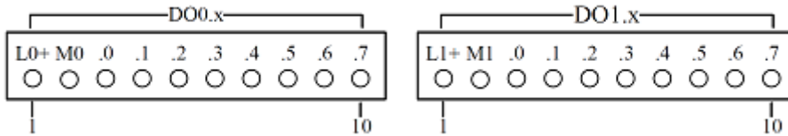
图 3-5 通用输出接口引脚定义
