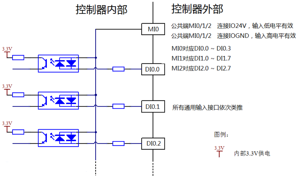
图 3-8 输入 I/O 接口内部电路
