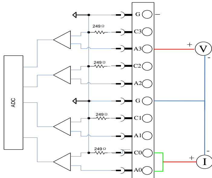
图 3-11 模拟量输入接线图
