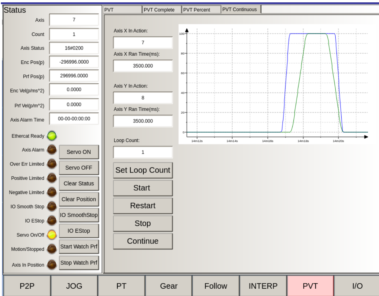
图 5-10 iBoxProDemo 界面 10
