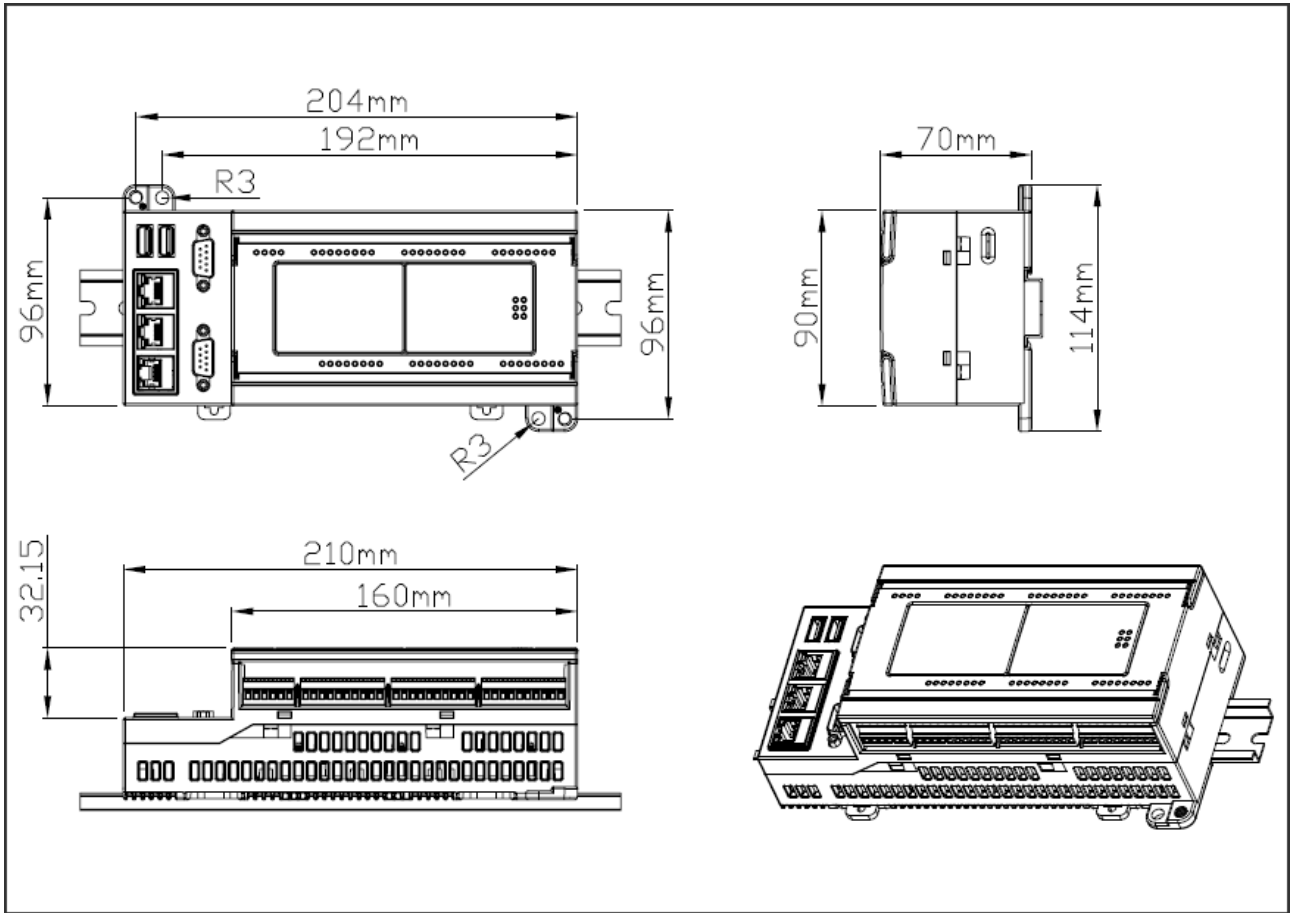
iDEABOX Pro 控制器尺寸图 单位(mm)
