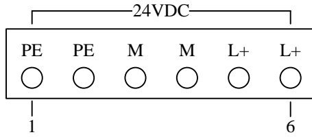
图 3-4 电源接口引脚定义
