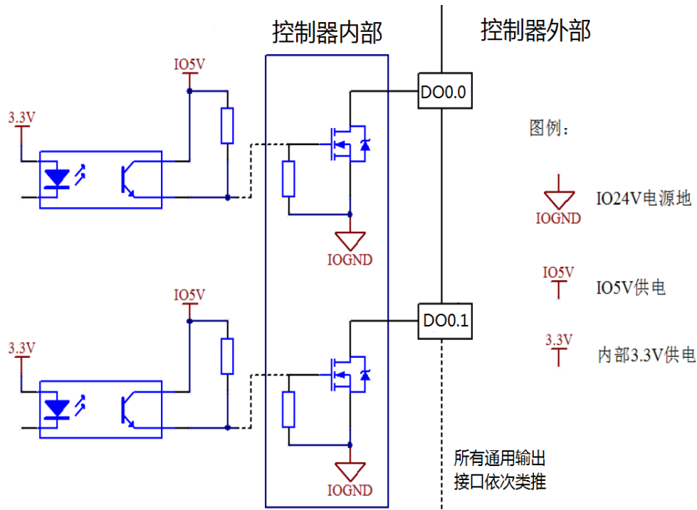
图 3-6 通用输出接口内部电路
