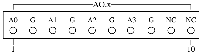
图 3-9 通用模拟量输出接口引脚定义
