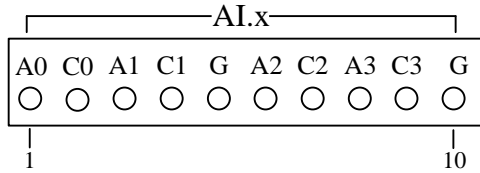
图 3-10 通用模拟量输入接口引脚定义
