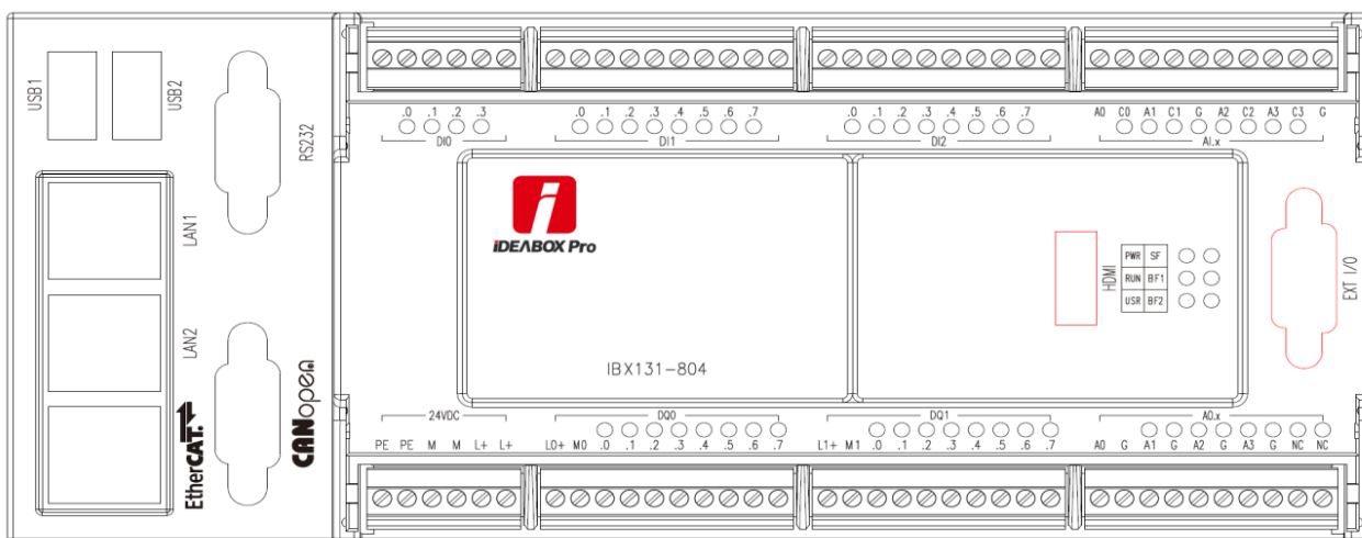
图 3-3 iDEABOX Pro 控制器接口示意图
