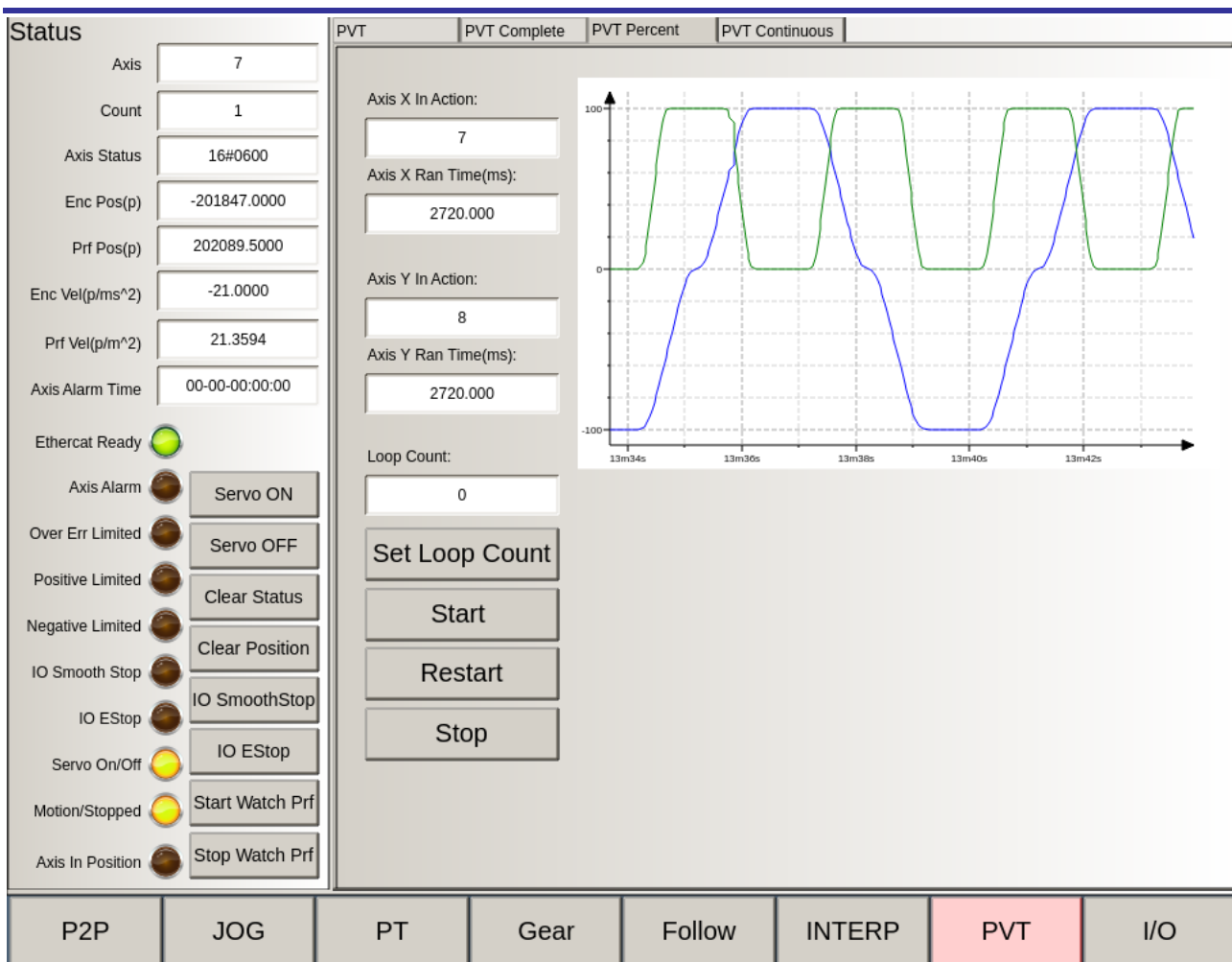
图 5-9 iBoxProDemo 界面 9
