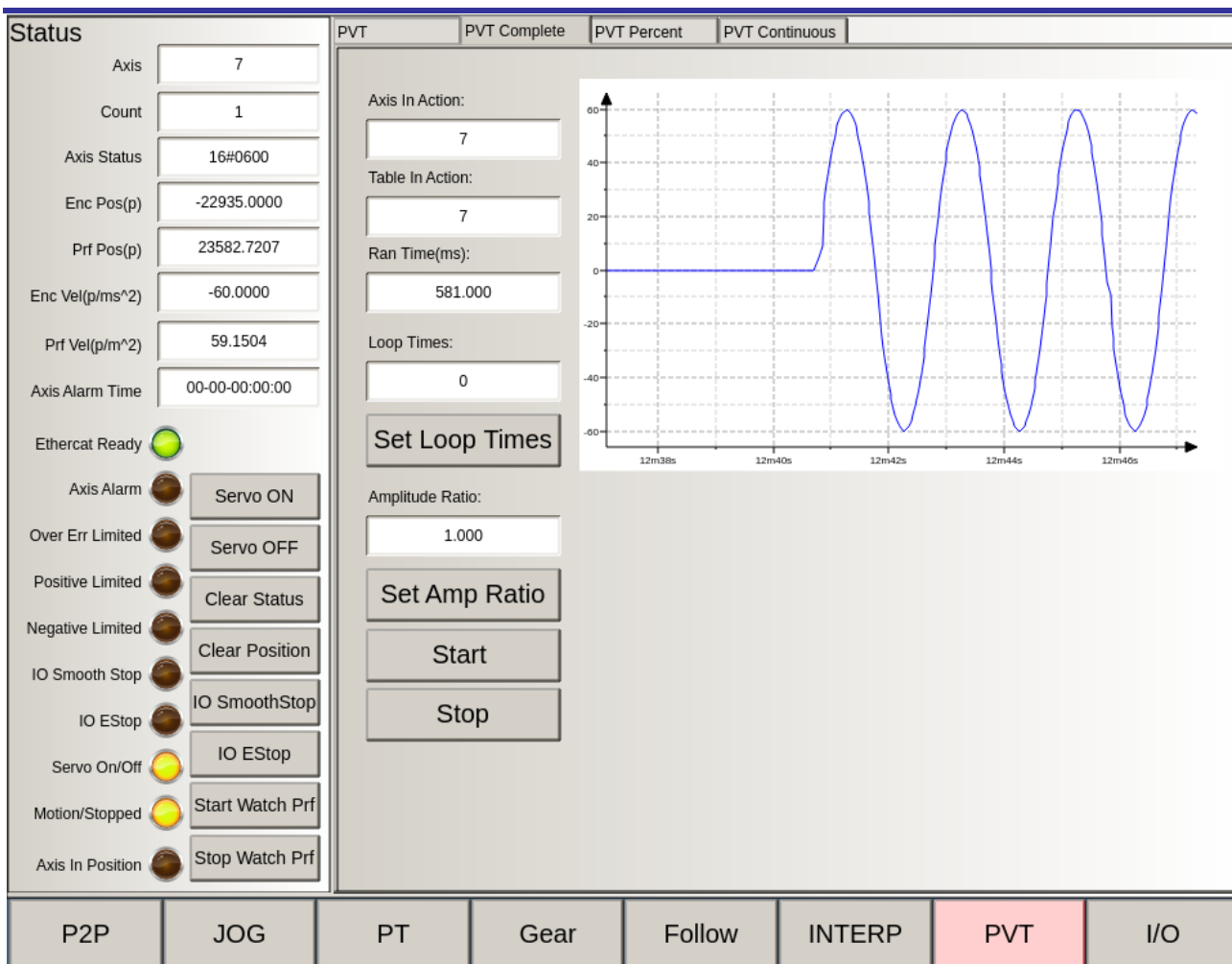
图 5-8 iBoxProDemo 界面 8
