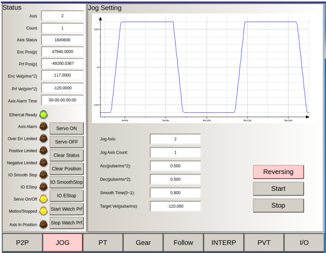
图 5-2 iBoxProDemo 界面 2
