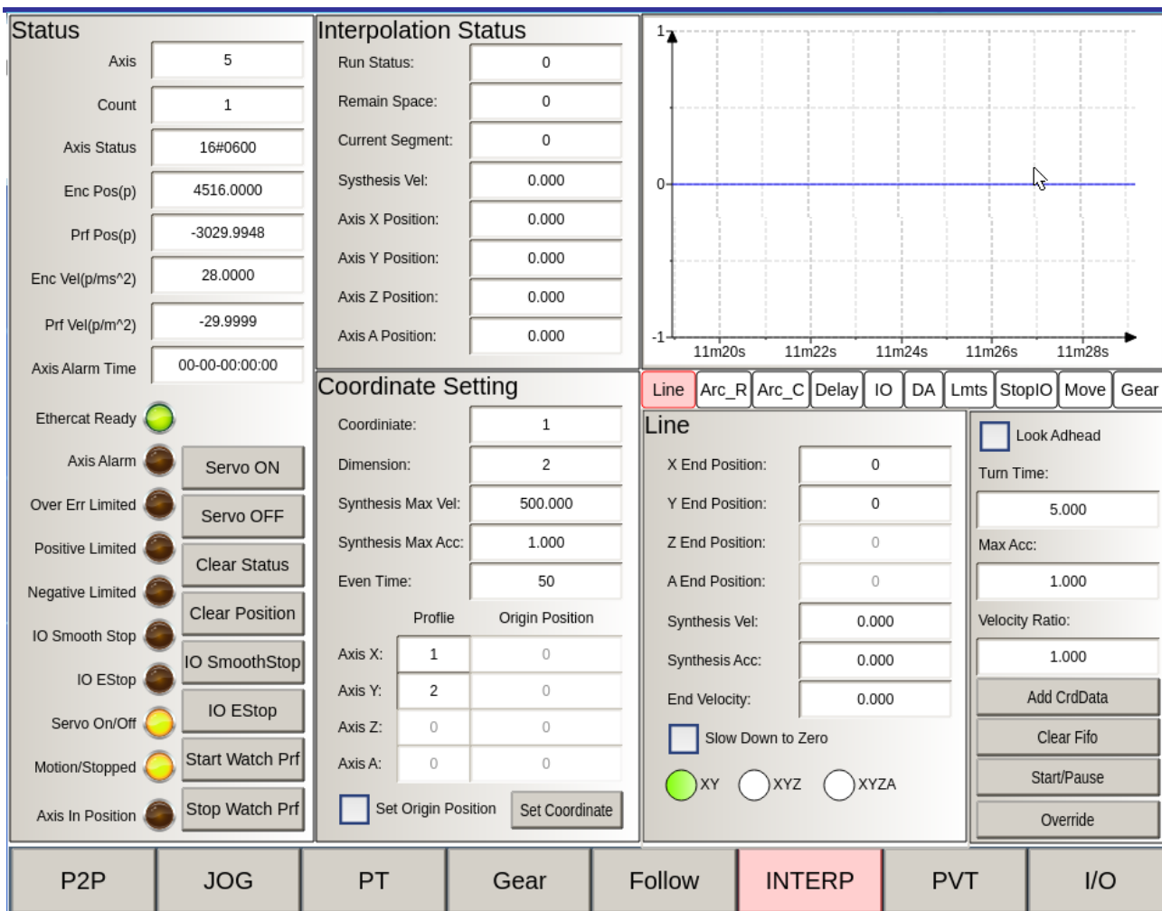
图 5-6 iBoxProDemo 界面 6
