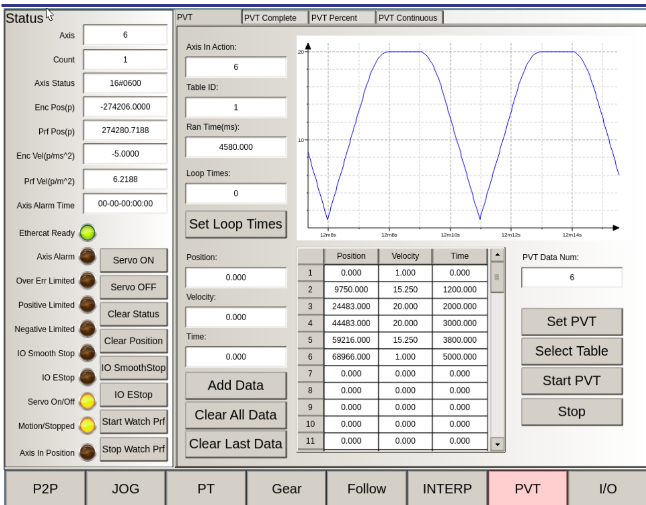
图 5-7 iBoxProDemo 界面 7
